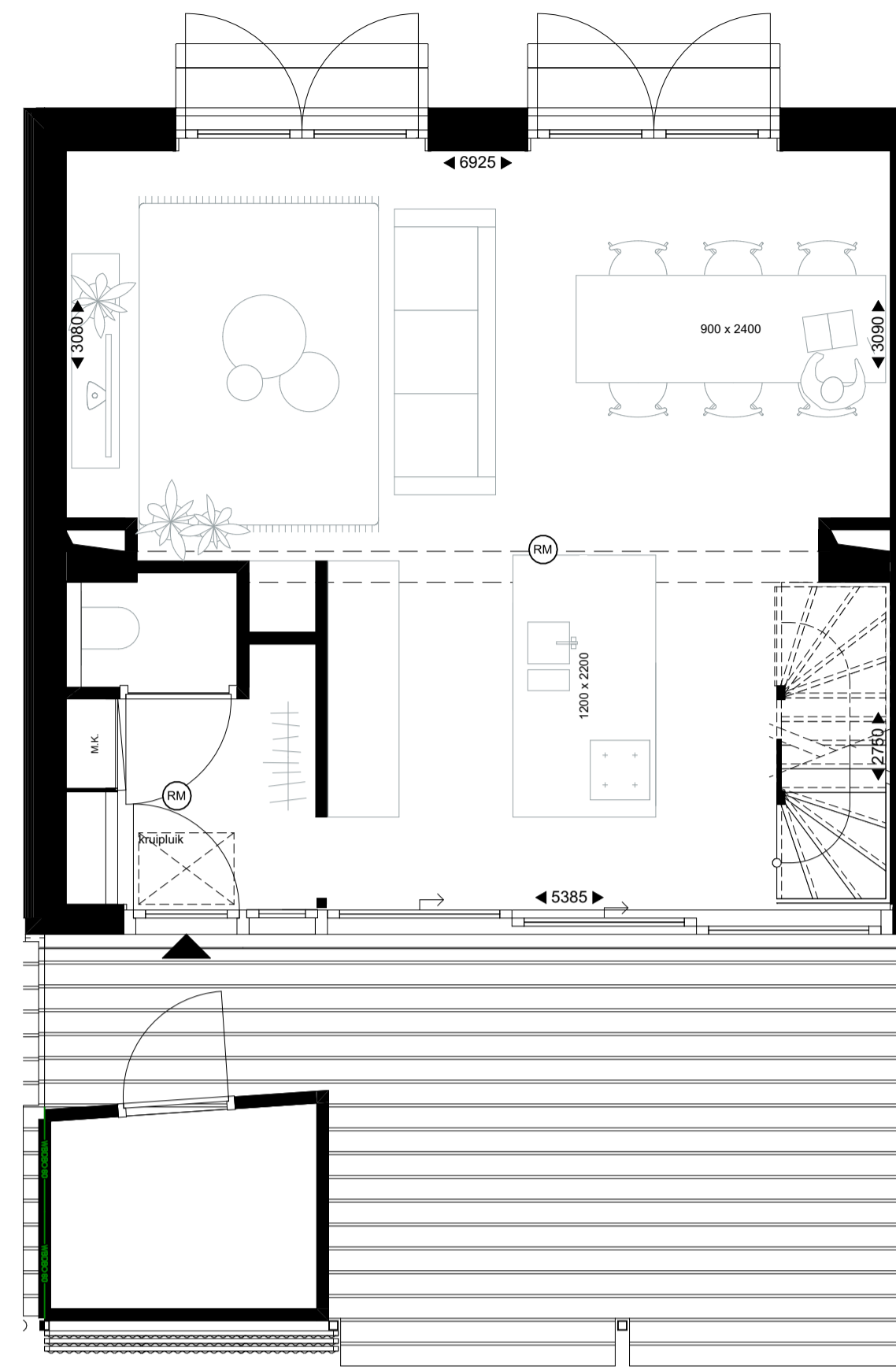
0. Begane grond 1:50
