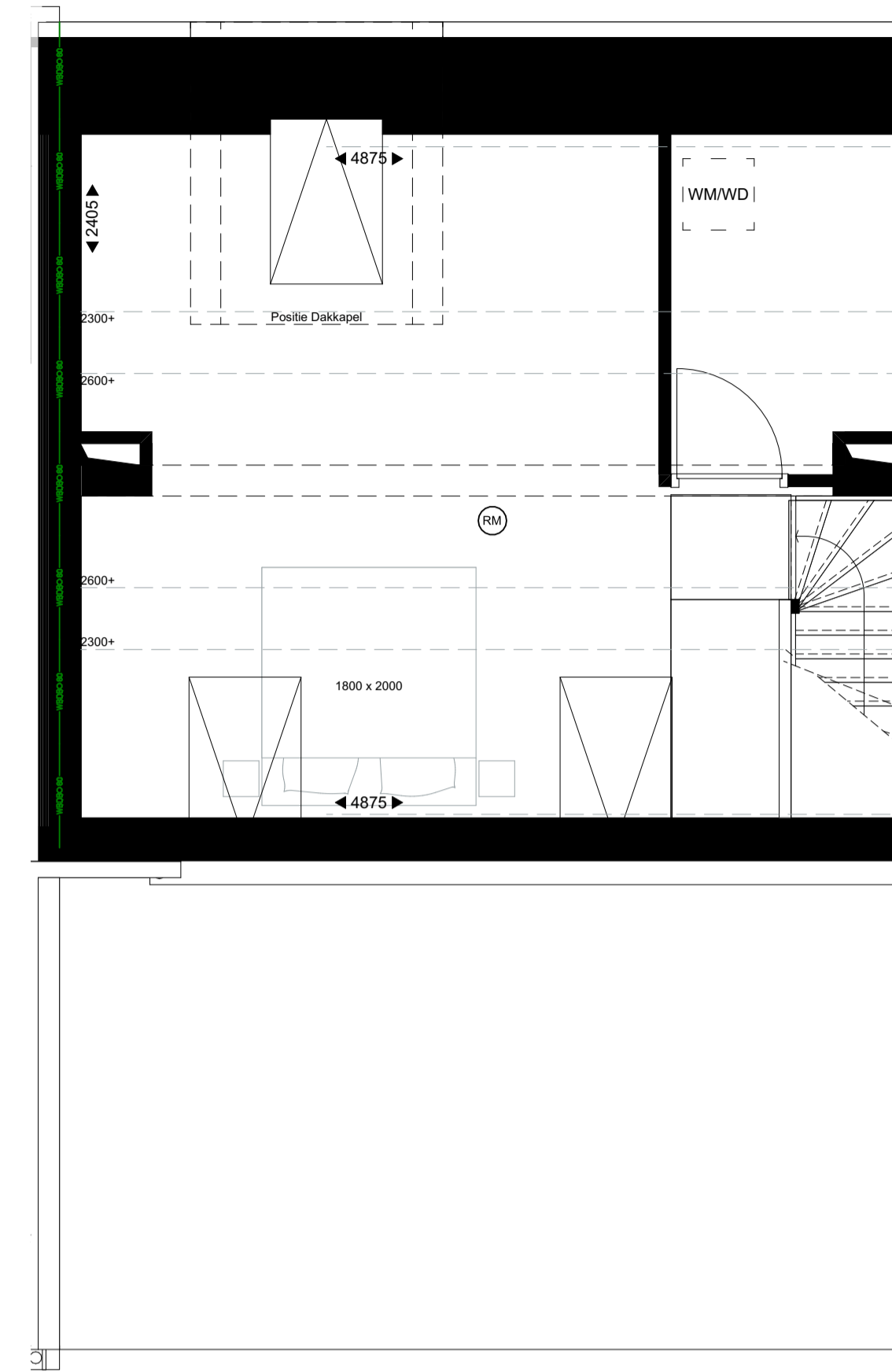
2. 2e verdieping 1:50
