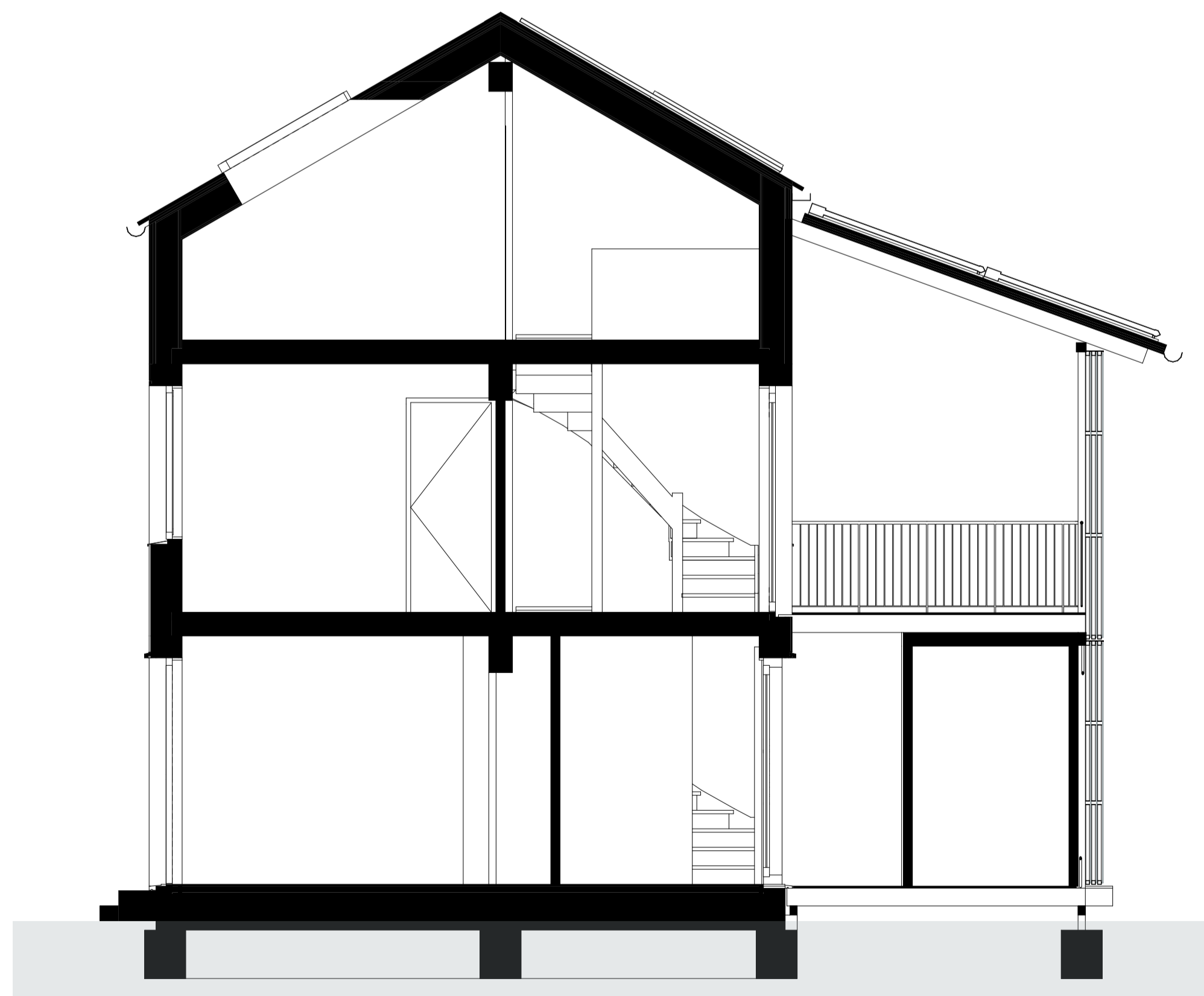
2_gD 1:50
