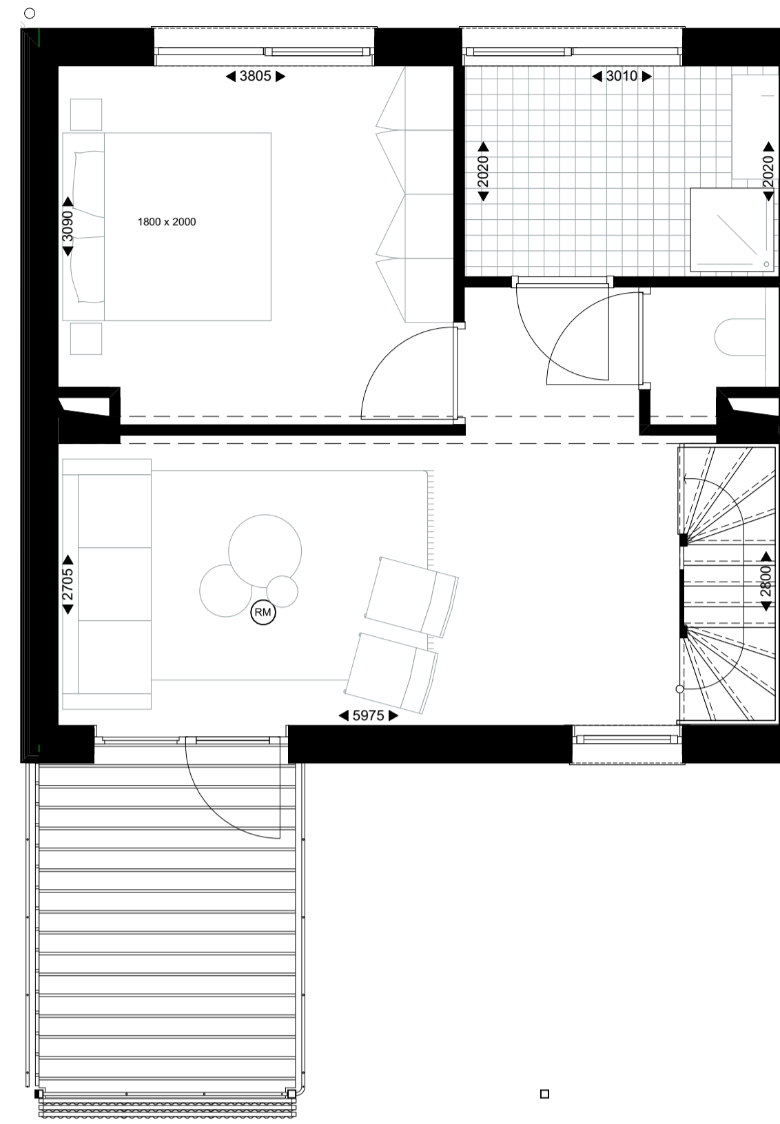
1. 1e verdieping 1:50
