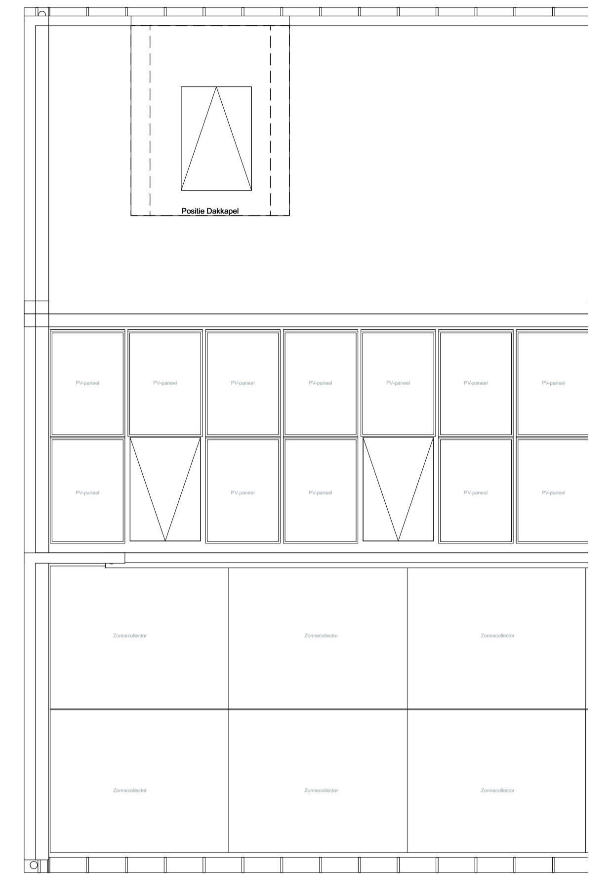
3. Nok / Dak 1:50
